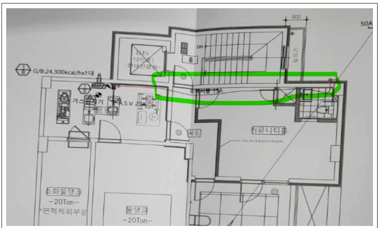
[그림 1] 건축물 내 은폐 배관 완공도면 점검구 미표기 예시
